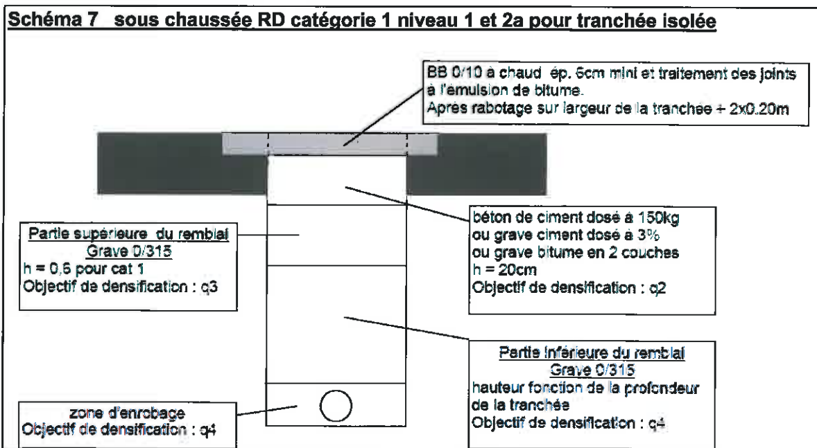
Schéma 7 sous chaussée RD catégorie 1 niveau 1 et 2a pour tranchée isolée (projet à faible impact type branchement particulier)
