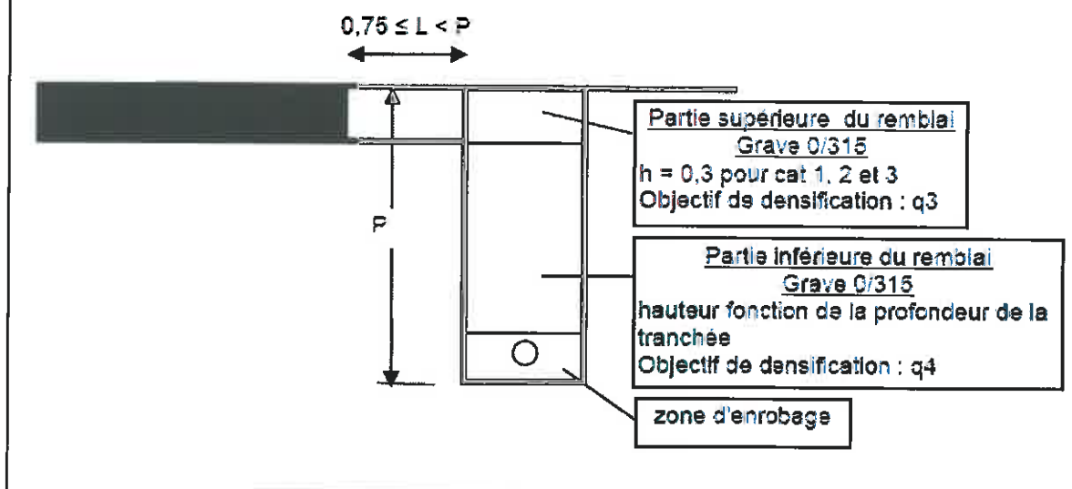
Schéma 6-1 tranchée sous accotement situé à une distance L du bord de chaussée comprise entre 0,75m et P (profondeur de la tranchée) pour RD des catégories 1, 2 et 3
