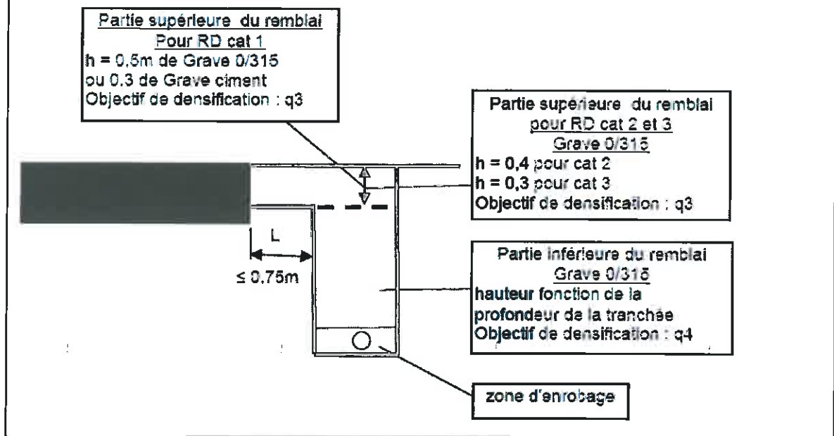
Schéma 7 sous chaussée RD catégorie 1 niveau 1 et 2a pour tranchée isolée (projet à faible impact type branchement particulier)
