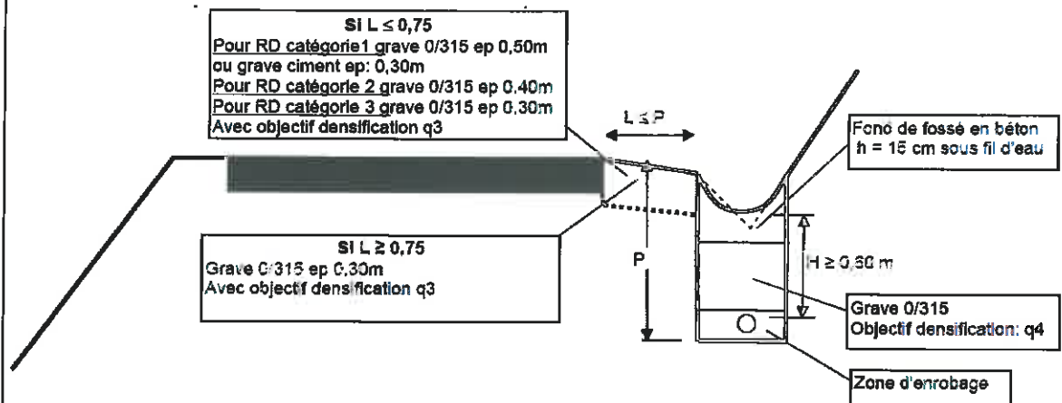
Schéma 5-2 tranchée sous fossé et proche du bord de chaussée des RD des catégories 1, 2 et 3
