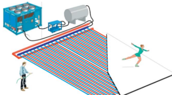
Schéma d'installation des entités constitutives pour un groupe froid de patinoire
