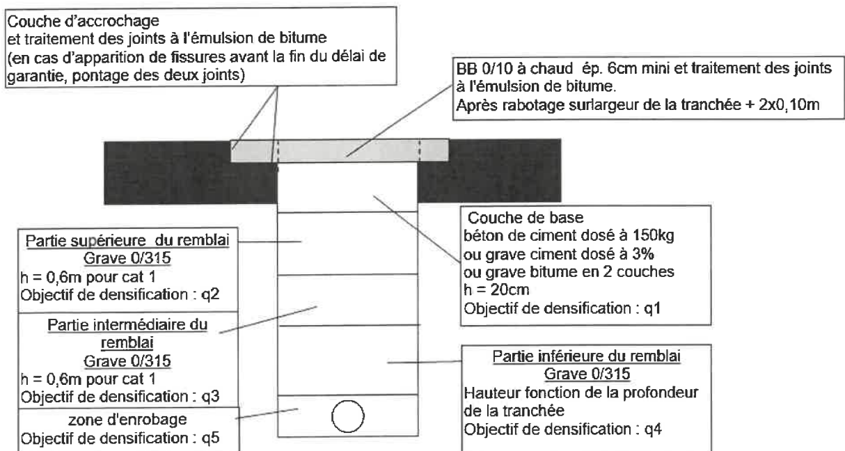
Schéma n°7 Tranchée isolée sous chaussée de toutes les RD (cat. 1, 2 et 3) (projet à faible impact type branchement particulier)
