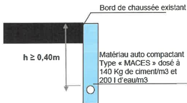
Schéma 3-2 tranchée étroite en rive de chaussée des RD des catégories 1, 2 et 3
