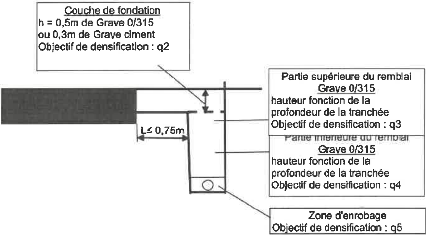
Schéma n°6-2 tranchée sous accotement située à une distance du bord de chaussée inférieure à 0,75m pour les RD des catégories cat.1, 2 et 3
