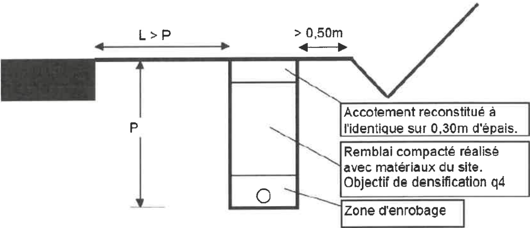
Schéma 4 tranchée sous accotement non revêtu, éloignée du bord de chaussée et du fossé des RD des catégories 1, 2 et 3
