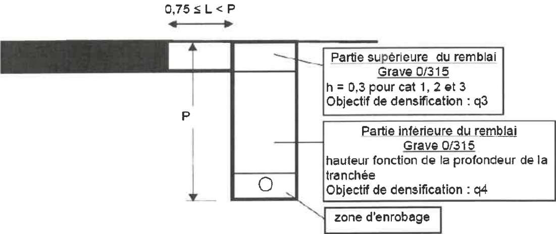
Schéma 6-1 tranchée sous accotement situé à une distance L du bord de chaussée comprise entre 0,75m et P (profondeur de la tranchée) pour RD des catégories 1, 2 et 3
