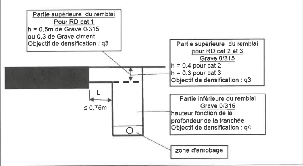
Schéma 6-2 tranchée sous accotement situé à une distance du bord de chaussée inférieure à 0,75 m pour RD des catégories 1, 2 et 3
